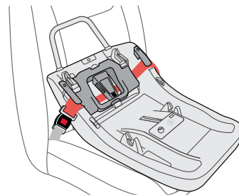
Instalación de la base con el cinturón para cadera
