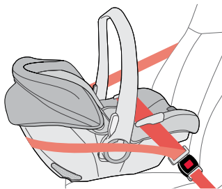
Instalación del cinturón para cadera y hombros con guía de cinturón europeo
